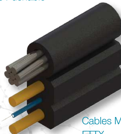
Cables Pushable
